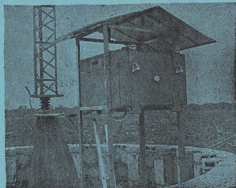
Unidad de sintonía del transmisor de 5.000 vatios instalada al piés de la torre-antena.
